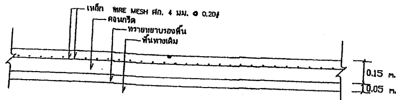
รายละเอียดถนนคอนกรีตเสริมเหล็ก
